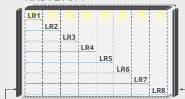
Bočne lajsne LRB Bočne lajsne sa LED napajanjem za plakare sa rasvetom ŠxVxD: 2,5x226x17,5cm
